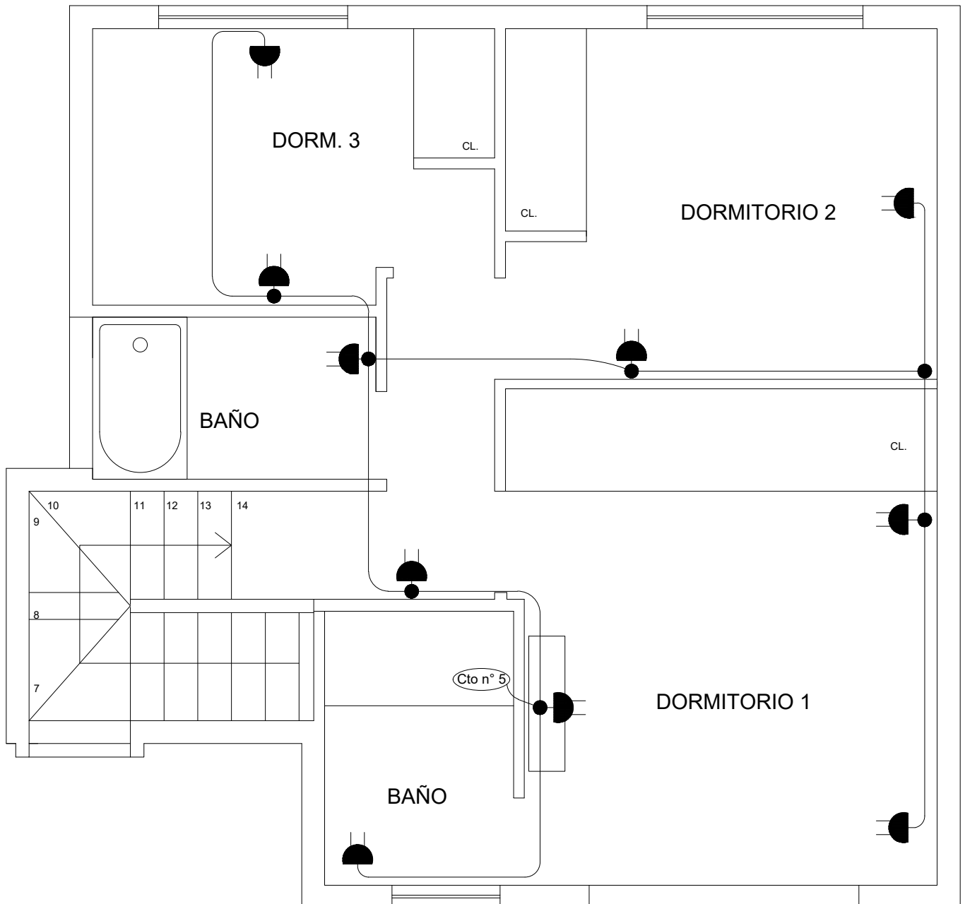
PLANTA ENCHUFES 2º PISO CASA TIPO AIRE
